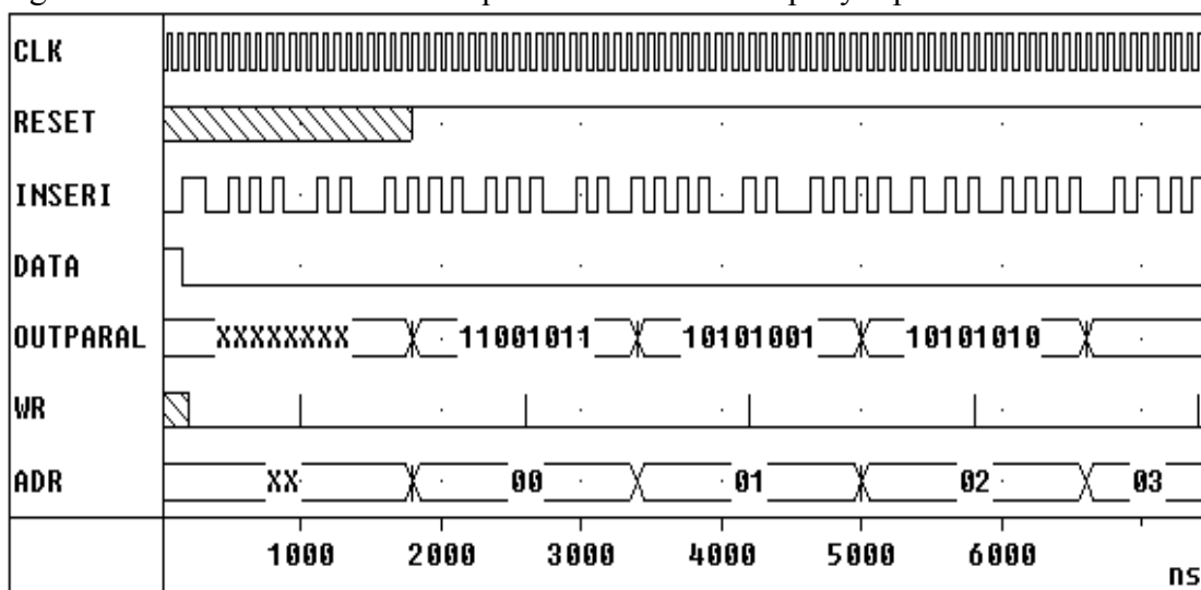
Gambar 9. Hasil Simulasi Modul Prekom
