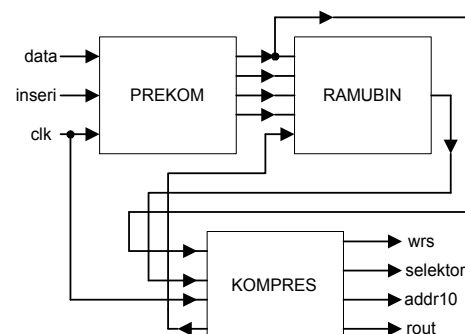
Gambar 3. Modul Penyusun Sistem Kompresi
