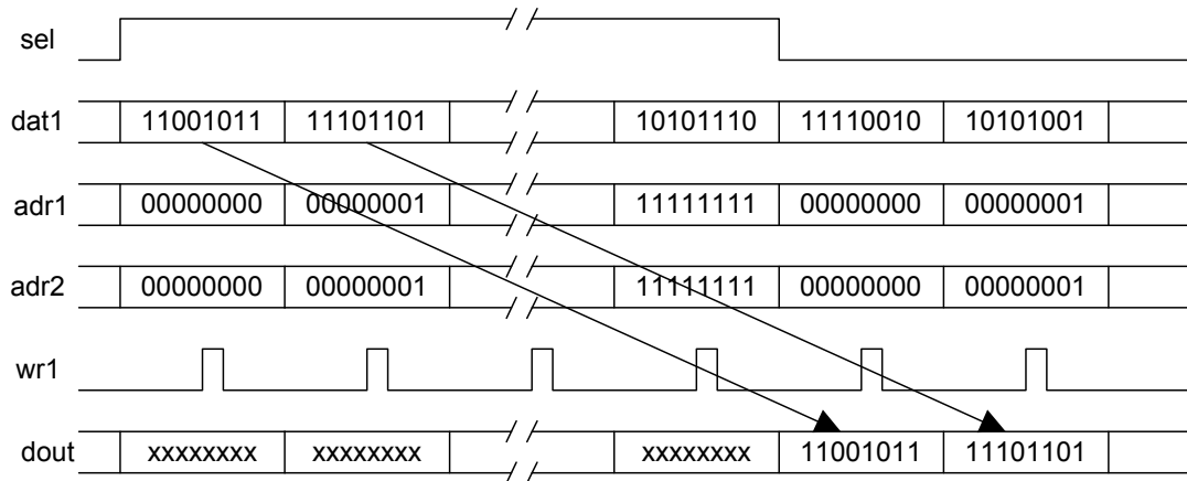
Gambar 5b. Diagram Waktu Ramubin
