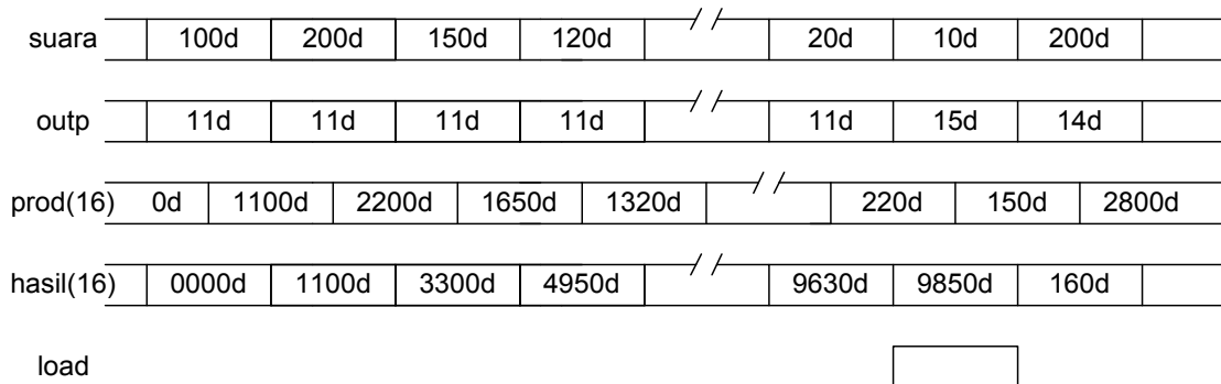
Gambar 8b. Diagram Waktu Transf
