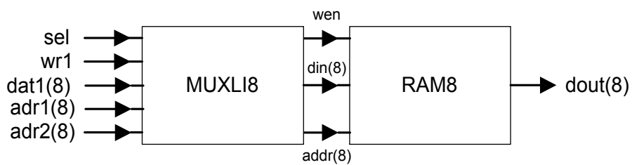
Gambar 5a. Modul Penyusun Ramubin
