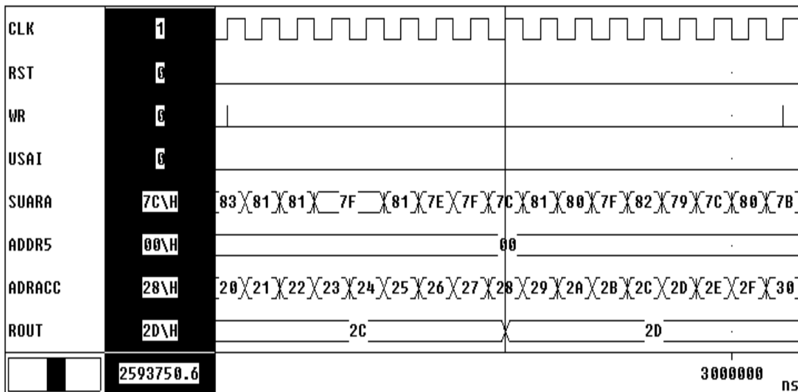
Gambar 12a Hasil Simulasi Fungsional Modul Kompres
