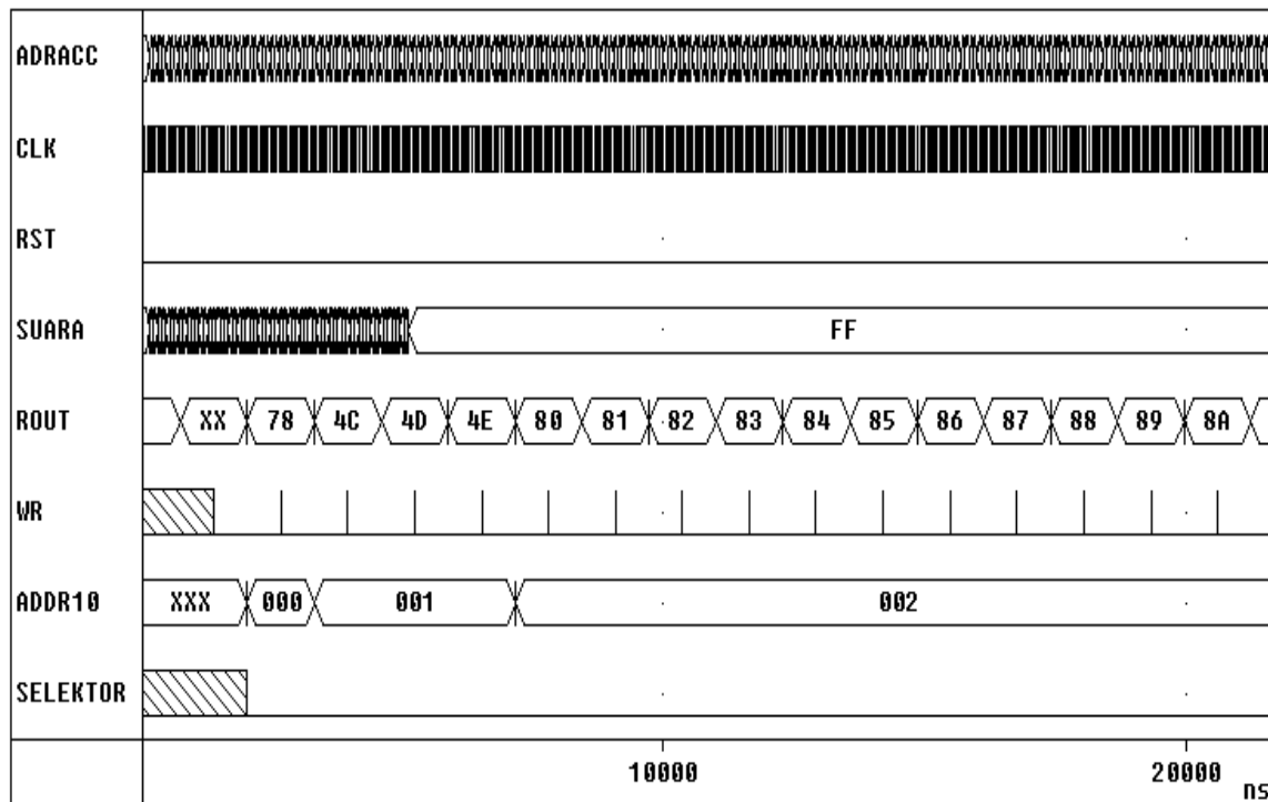
Gambar 11 Hasil Simulasi Modul Kompres
