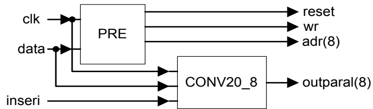
Gambar 4a. Modul Penyusun Prekom
