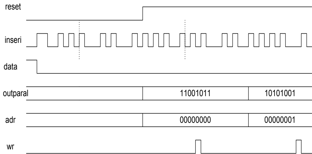
Gambar 4b. Diagram Waktu Prekom
