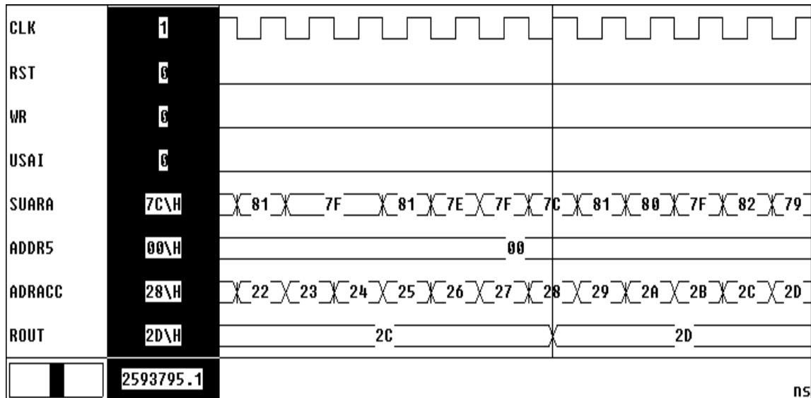
Gambar 12b Hasil Simulasi Pewaktuan Modul Kompres
