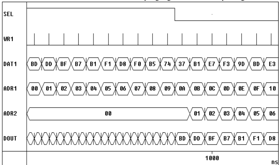
Gambar 10 Hasil Simulasi Modul Ramubin
